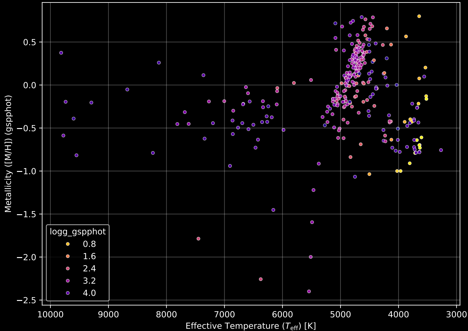
APOGEE DR17 Field: [030+04] Stellar Population Parameters (n= 315)
